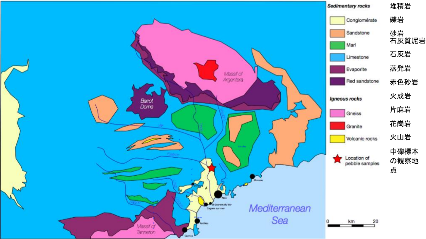
図4：Var谷とその支流地域の単純化した地質図。図3の中礫の写真は、赤い星印が付いた場所から採取したもの。
