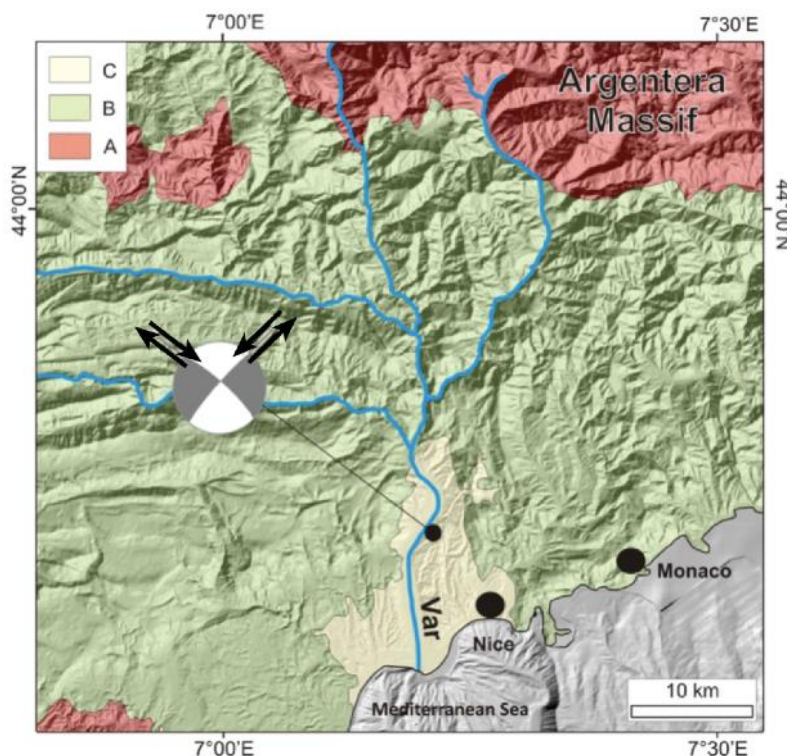
図14 Var谷の構造図で、最近のある地震でできたある断層沿いの相対的な動きを示している（塗色された部分のある円。円内の2本の線は、見出されていない仮想の断層の方向を、矢印は可能性のある断層それぞれの相対運動を示している）。凡例：A 結晶質の基盤岩、B 中生代の堆積岩の分布、C 鮮新世～第四紀堆積物 地図に示した震央の位置の近くに、図13の断層面が観察された。
