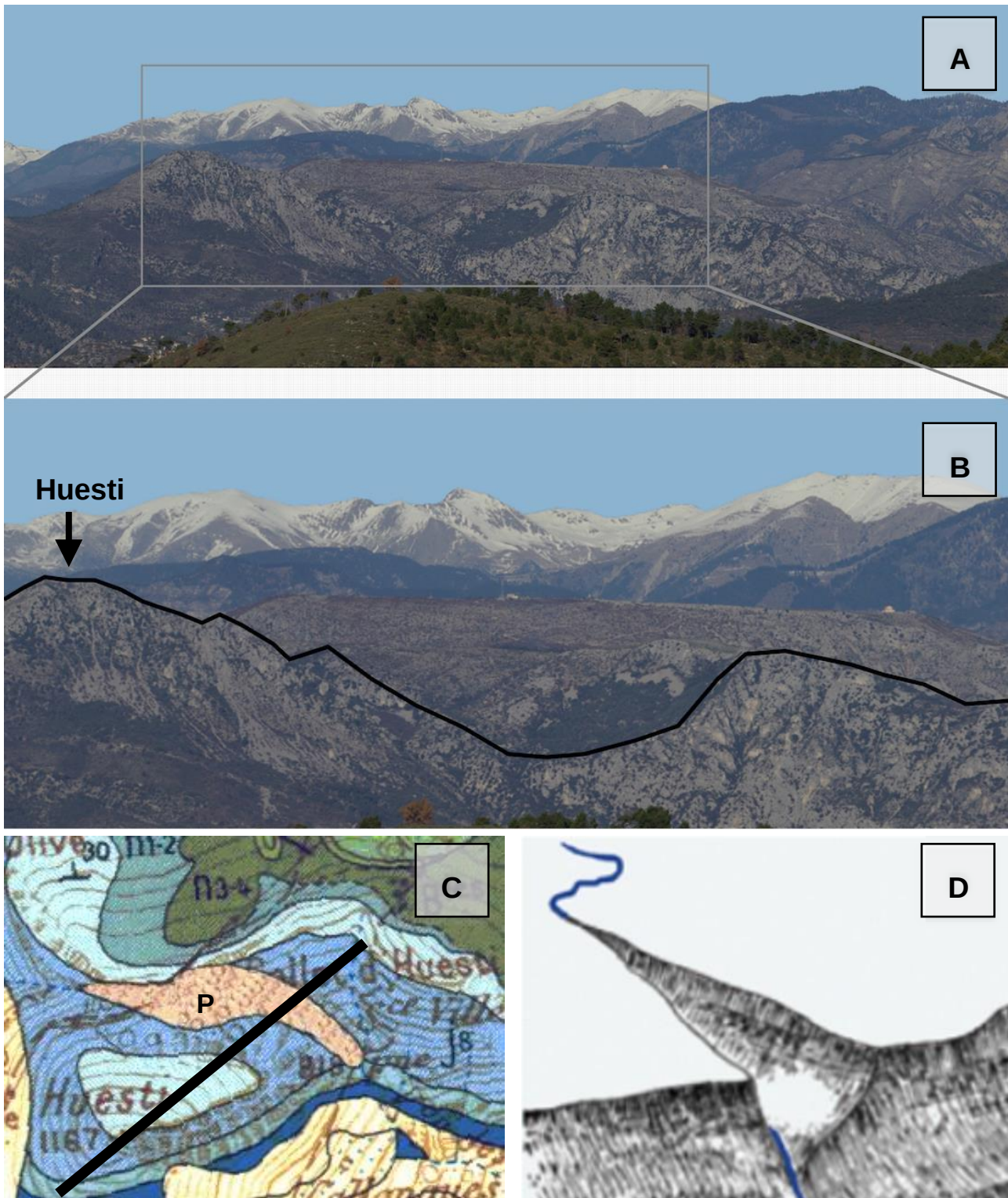
図 16: (A) Var 谷の北側の南アルプスの展望; (B) Mount Huesti (標高1167 m) の展望; (C) Mount Huestiの地質図。黒い太線は図(B)の写真が写している範囲を表している。地質図中の色は岩石の年代を示している: 青系統色-ジュラ紀, 緑系統色-白亜紀, オレンジ (地図中のp) -鮮新世, 黄色-第四紀 (斜面崩壊堆積物); (D) 峡谷のスケッチ
