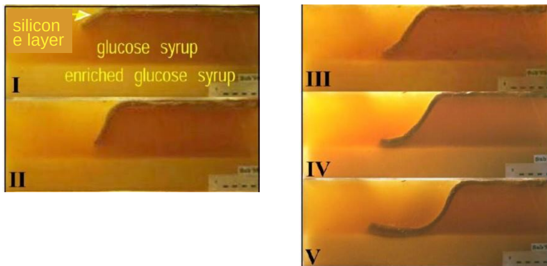
図18 : Claudio Faccenna (University of Rome, 2003) の収束無しの沈み込み実験結果。IからVは実験で撮影された連続写真。Silicone layer: シリコーン層, glucose syrup: グルコースシロップ, enriched glucose syrup: グルコース濃度の高いシロップ
