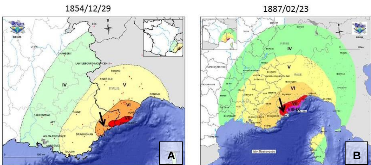
図12: 1854年 (A)と1887年 (B)の地震における等震度線図。色付けされた領域は、同じ震度で揺れた場所を示している。ヴァール谷は黒矢印で示されている。
