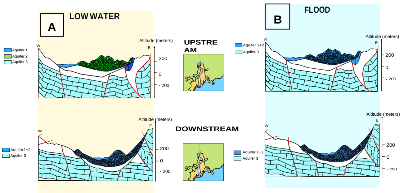
図8 Var谷における、(A) 水位が低いとき（乾季）、(B) 雨季における断面図
