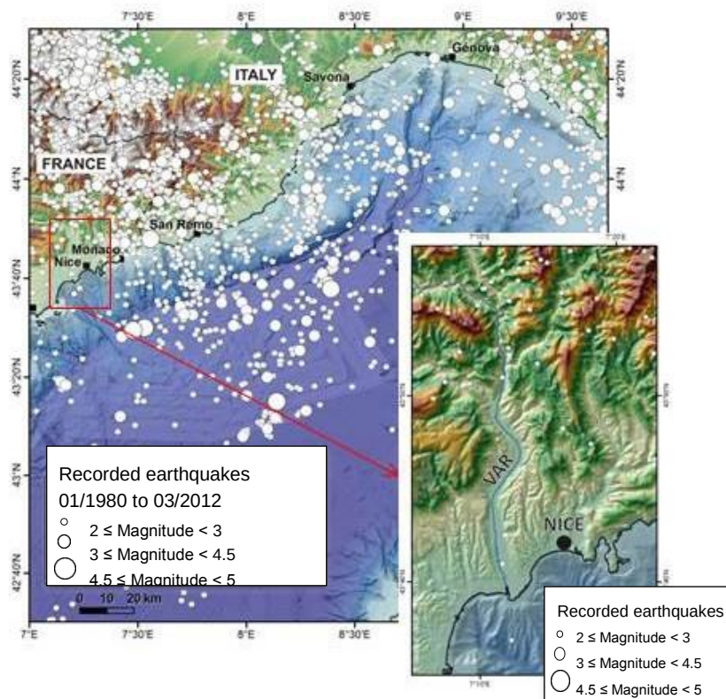
図9： この地域の震源図（地震計による震央の場所）とヴァール谷（対象エリア）の拡大図。震源の深さは30kmを超えない。
